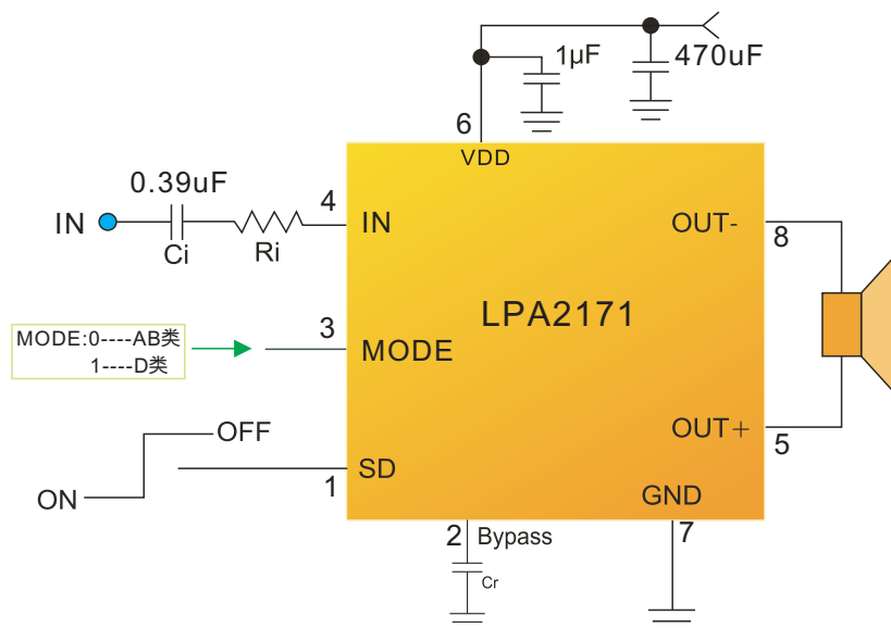
LPA2171应用电路图
