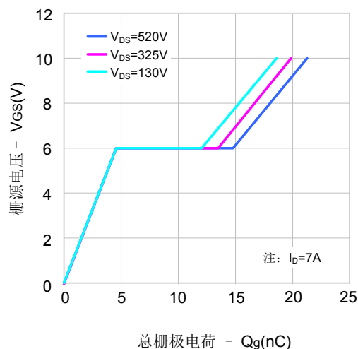
图6. 电荷量特性
