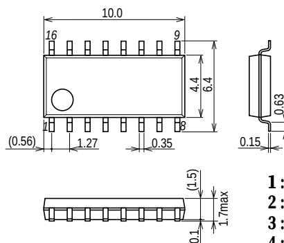
外形図 2198 (unit : mm)
